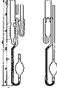
المسقط الرأسى شكل رقم ( ١٠ ) مقياس اللزوجة من نوع ( لانترز - زيتفوس )
