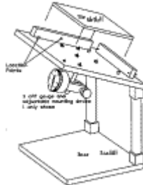
شكل رقم ( ٢٤ ) جهاز فحص الانفتال والتقعر في البلاط
